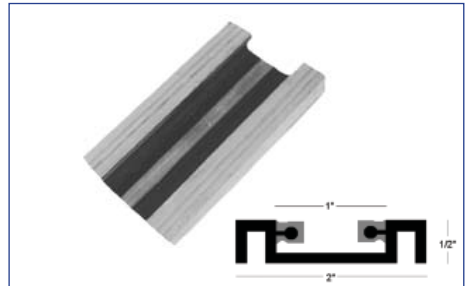
C0367 Pin Guide Bottom Track
